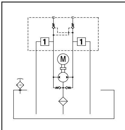
Schema idraulico
