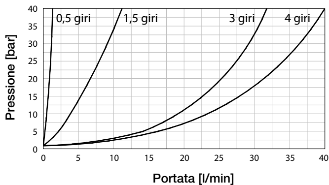
DIAGRAMMA PERDITE DI CARICO
