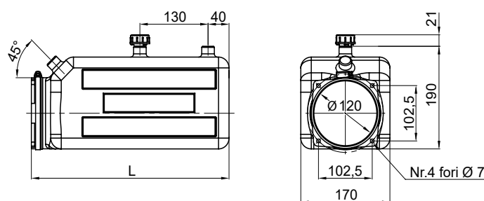
Serbatoi 8,0 / 12 Lt. (con 3 fori)
