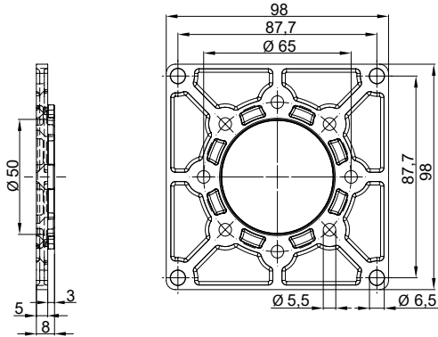
Flangia di adattamento
