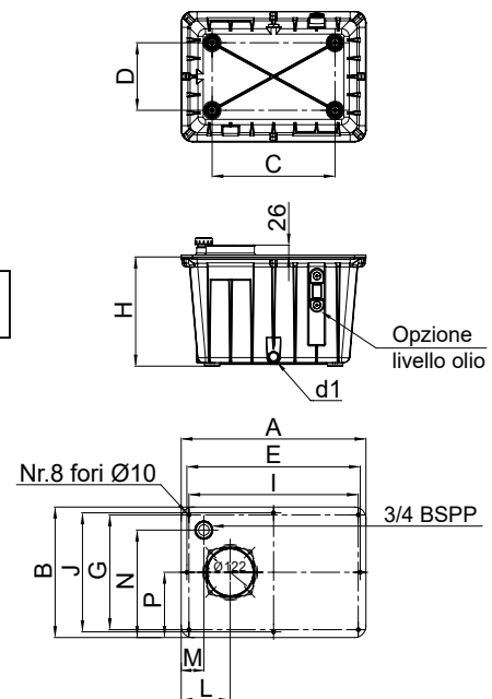
Serbatoi 16 / 25 Lt.
