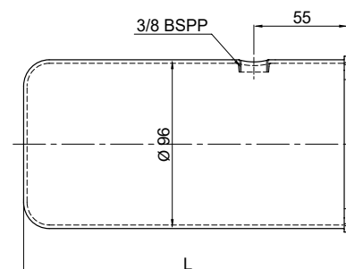
Serbatoi Ø96
