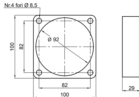
Collare CL05
