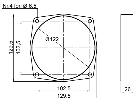
Collare CL10
