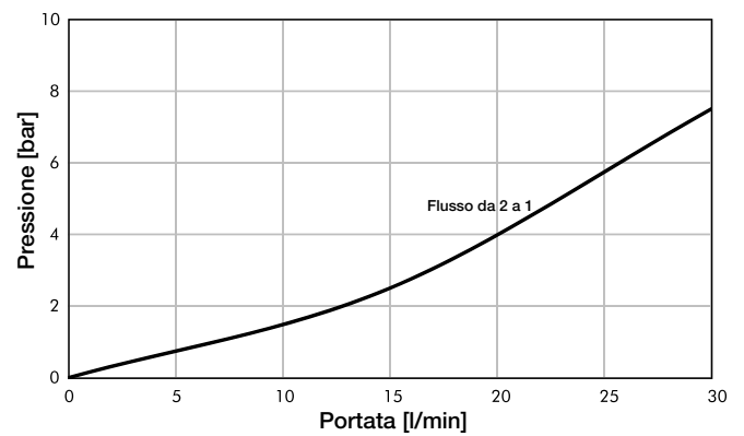
Elettrovalvola VSB
