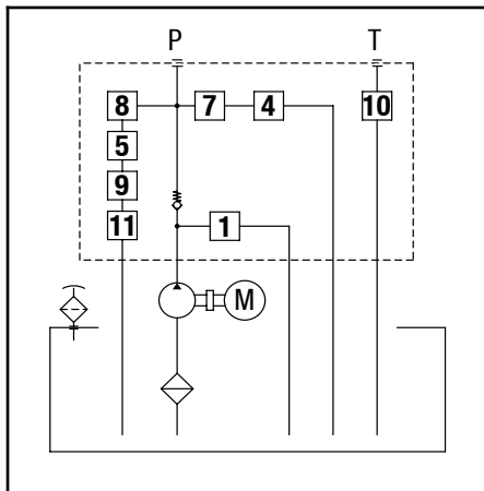
Schema idraulico
