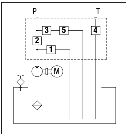
Schema idraulico
