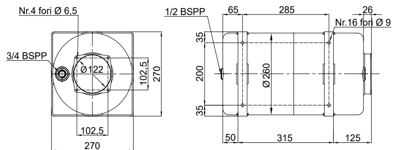
Serbatoio Ø260 verticale
