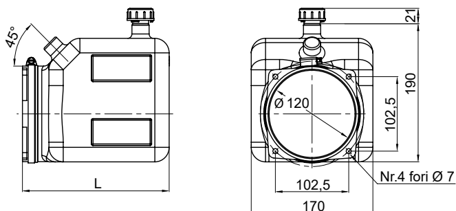
Serbatoi 1,5 / 3,0 / 5,0 Lt. (con 2 fori)
