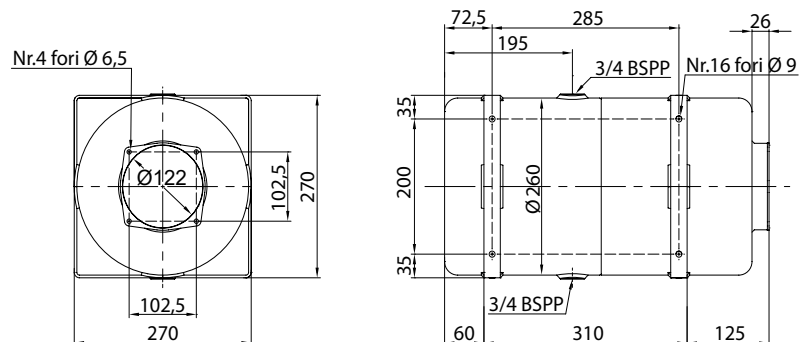
Serbatoio Ø260 orizzontale
