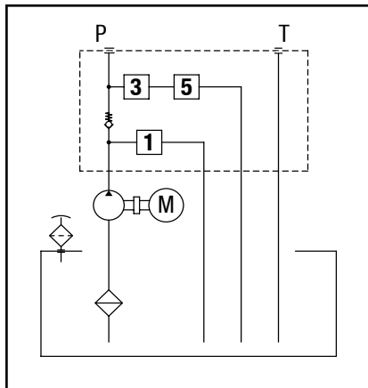
Schema idraulico
