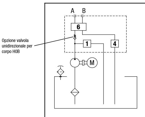
Schema idraulico
