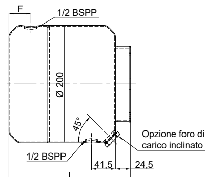
Serbatoi Ø200
