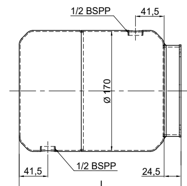
Serbatoi Ø170
