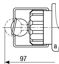
Comando di emergenza manuale N3 con detent
