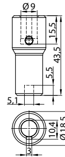
Giunto
