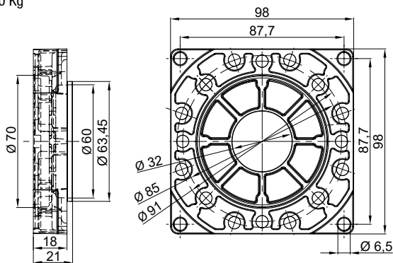
Flangia di adattamento
