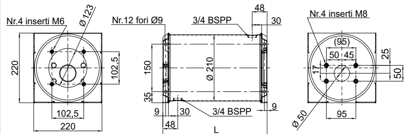
Serbatoi Ø210
