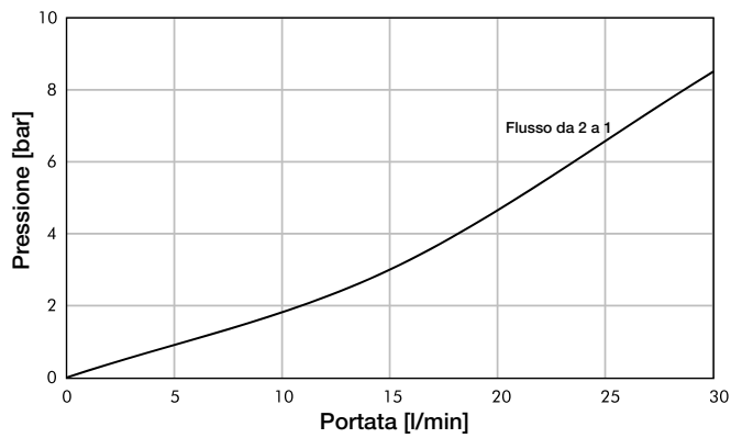
Elettrovalvola VSA
