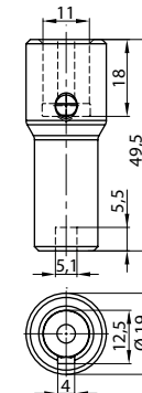
Giunto
