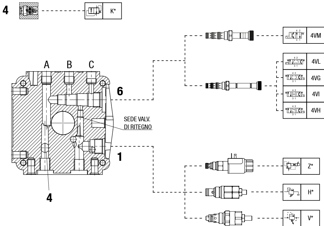
Schema idraulico
