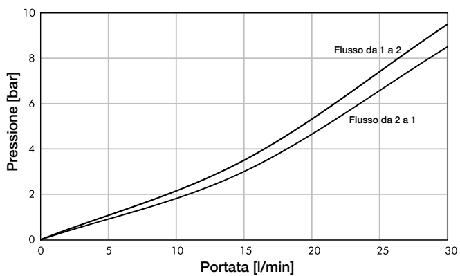
Elettrovalvola VSC
