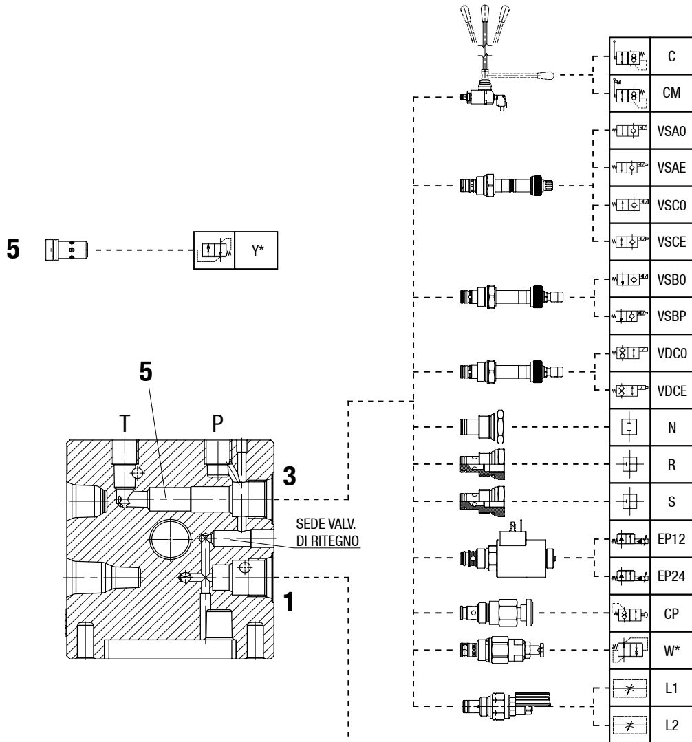
Schema idraulico
